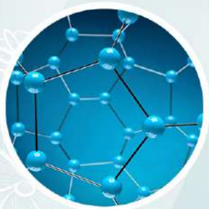
FULLERENE
